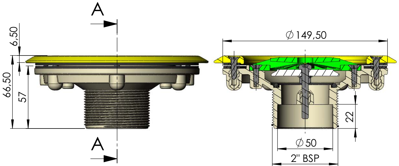
SECCIÓN A-A
